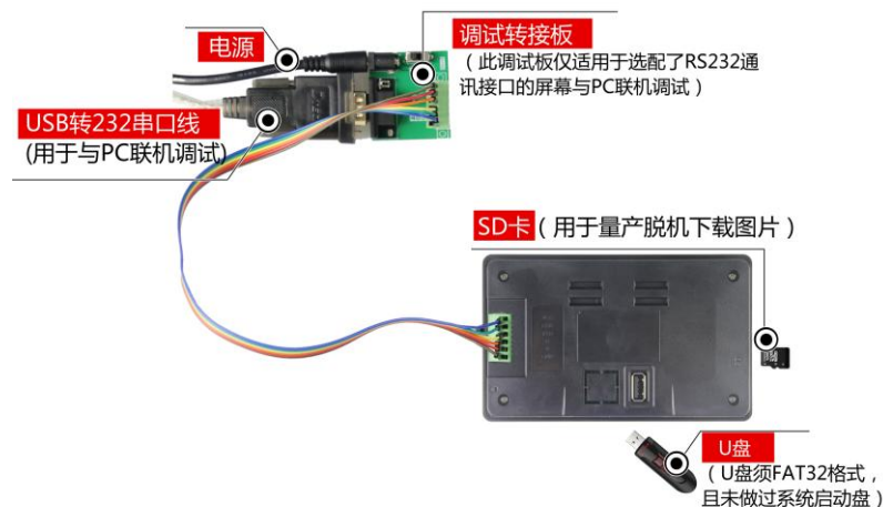
图 1-4 RS232 调试图
