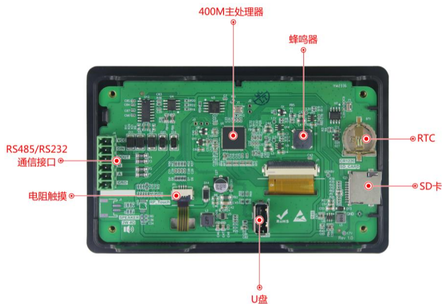
图 1-2 硬件配置图
