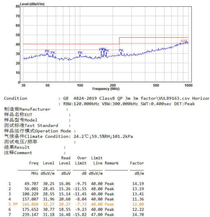
图 6-6 RE 测试垂直方向
