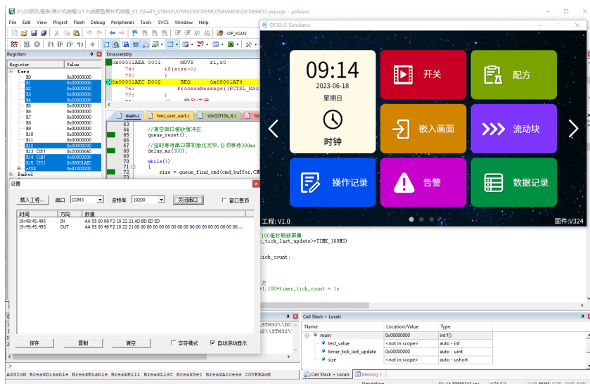
图 8-3 Keil 开发环境与“HMI 模拟器”绑定调试
