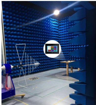
图 6-4 RE 测试图
