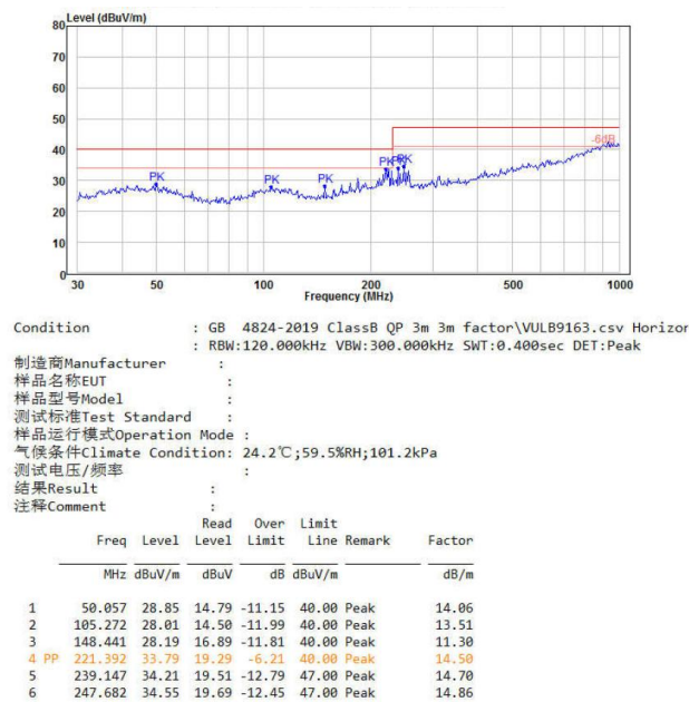
图 6-5 RE 测试水平方向
