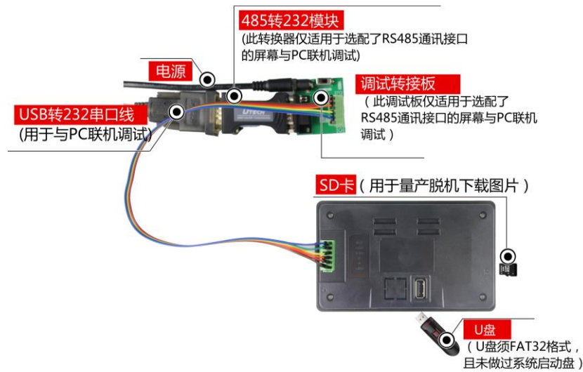
图 1-3 RS485 调试图
